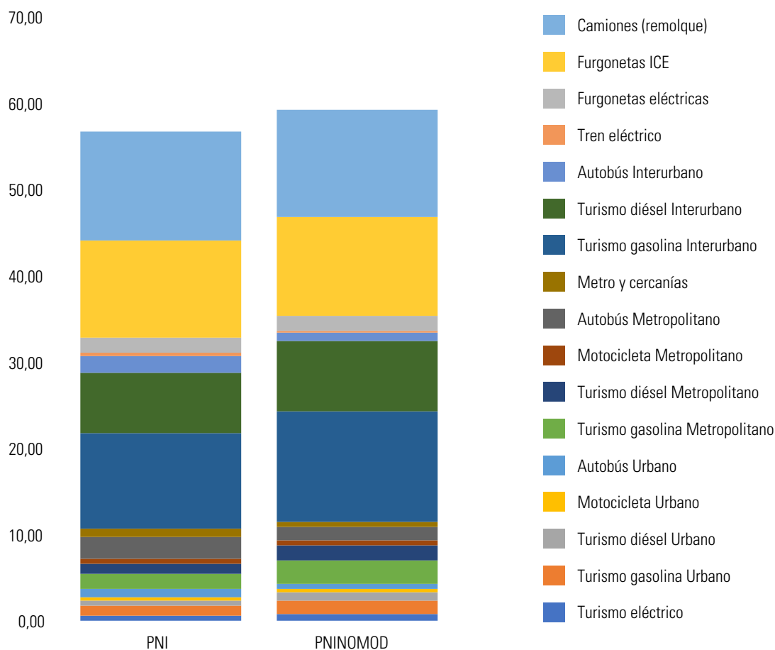
Gráfico 18. Sensibilidad PNI – PNINOMOD. Millones de toneladas de CO 2
